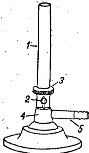
Bunsen-égő
